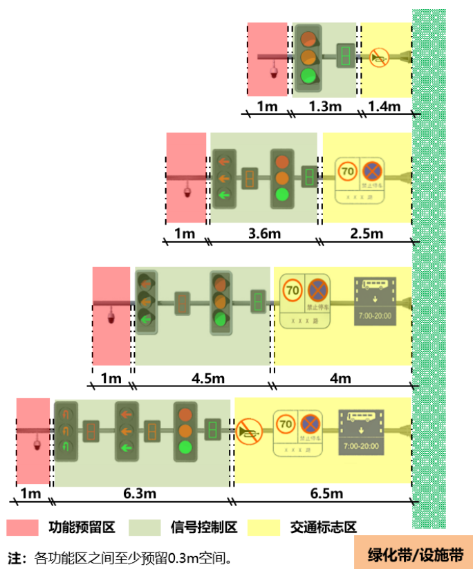
图 4.1.7-1 杆件功能预留区域示意图 1
