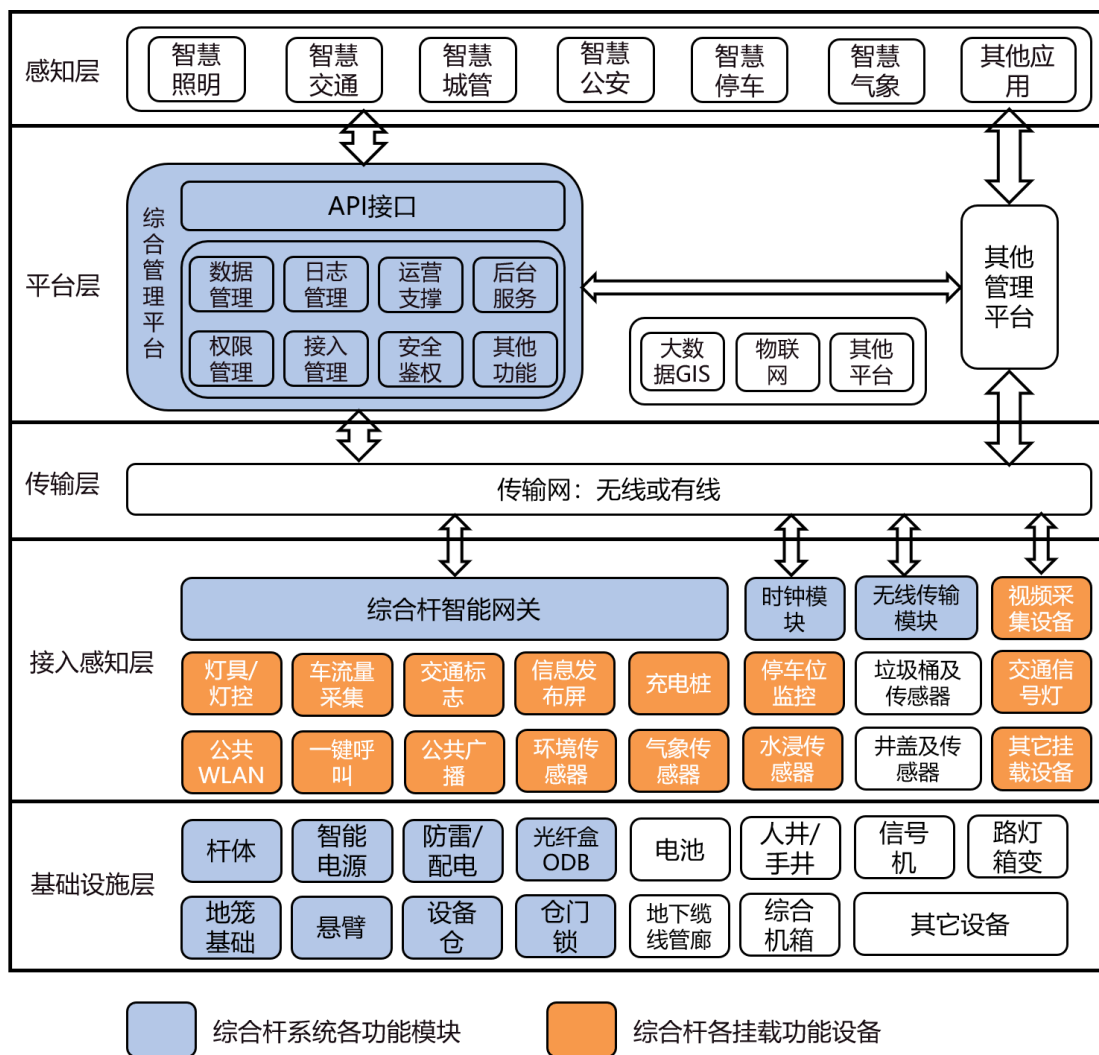
图 7.1.1 综合管理平台总体架构示意图
